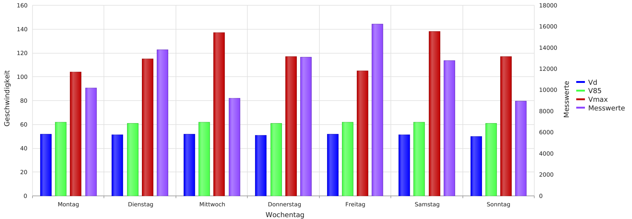
2023_04_20-05_03 Essel K105 Richtung Ortskern Vd, V85, Vmax, Anzahl der Messwerte vs. Wochentag
