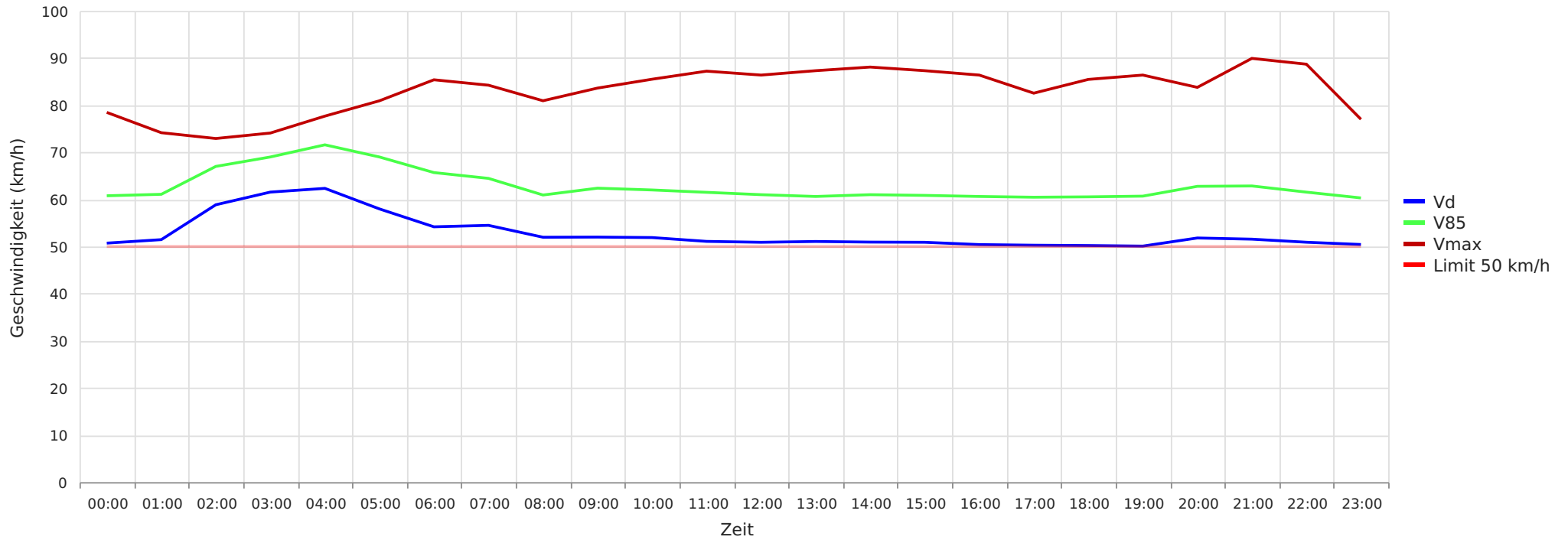
2023_04_20-05_03 Essel K105 Richtung Ortskern Vd, V85, Vmax vs. Uhrzeit
