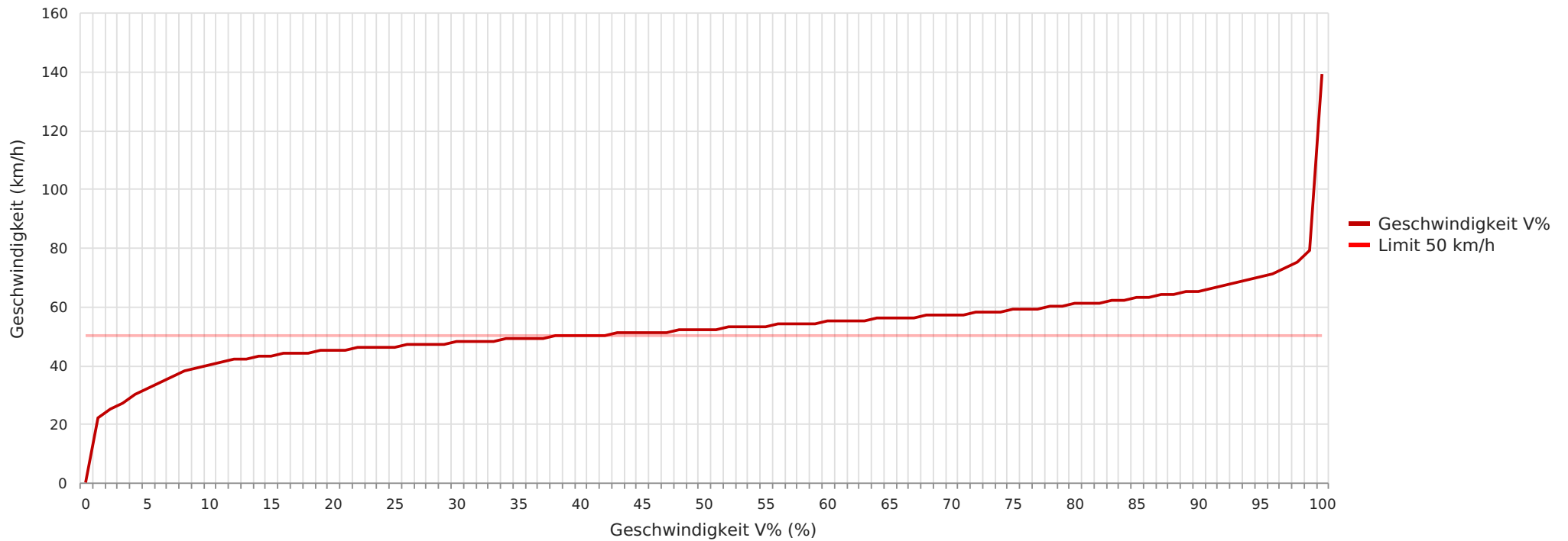
2023_04_20-05_03 Essel K105 Richtung Ortskern Geschwindigkeit vs. prozentueller Anteil an Messwerten
