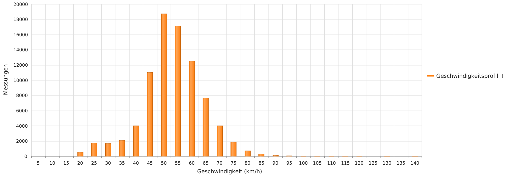
2023_04_20-05_03 Essel K105 Richtung Ortskern Anzahl der Messwerte vs. Geschwindigkeit
