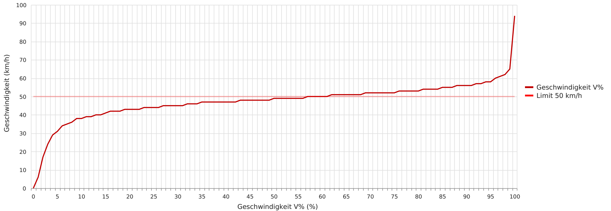
2023_11_12-12_25 Hope Hauptstraße Richtung Grindau Geschwindigkeit vs. prozentueller Anteil an Messwerten
