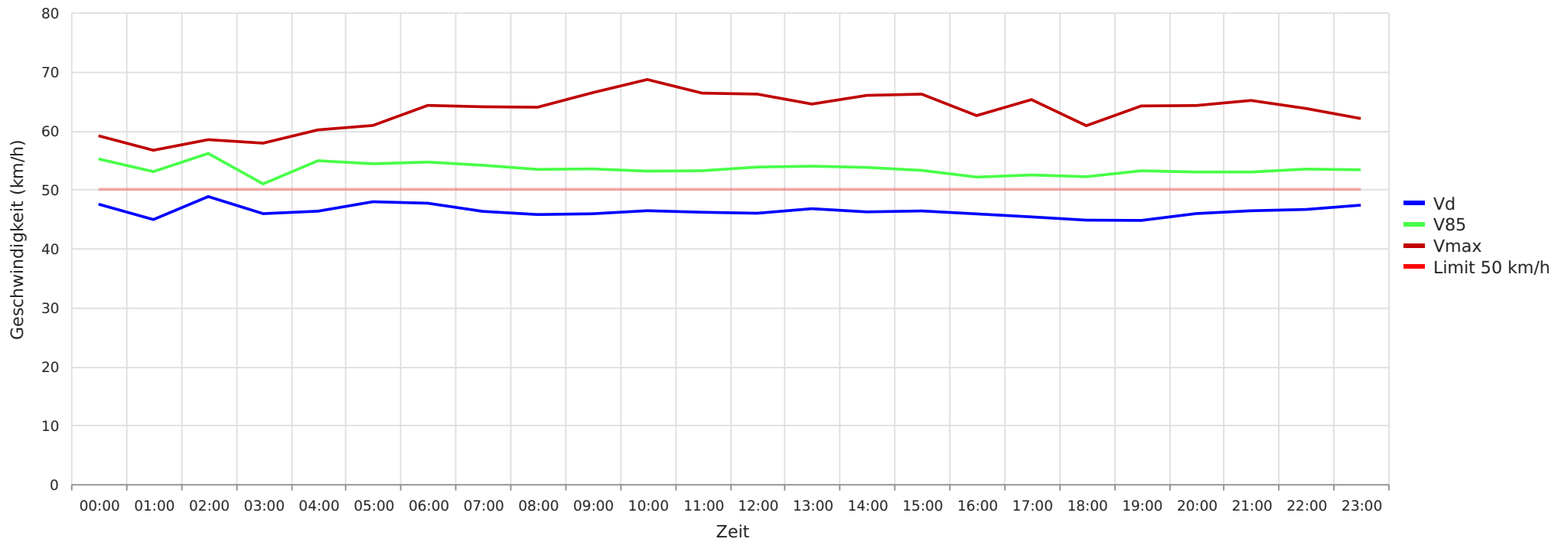
2023_11_12-12_25 Hope Hauptstraße Richtung Grindau Vd, V85, Vmax vs. Uhrzeit
