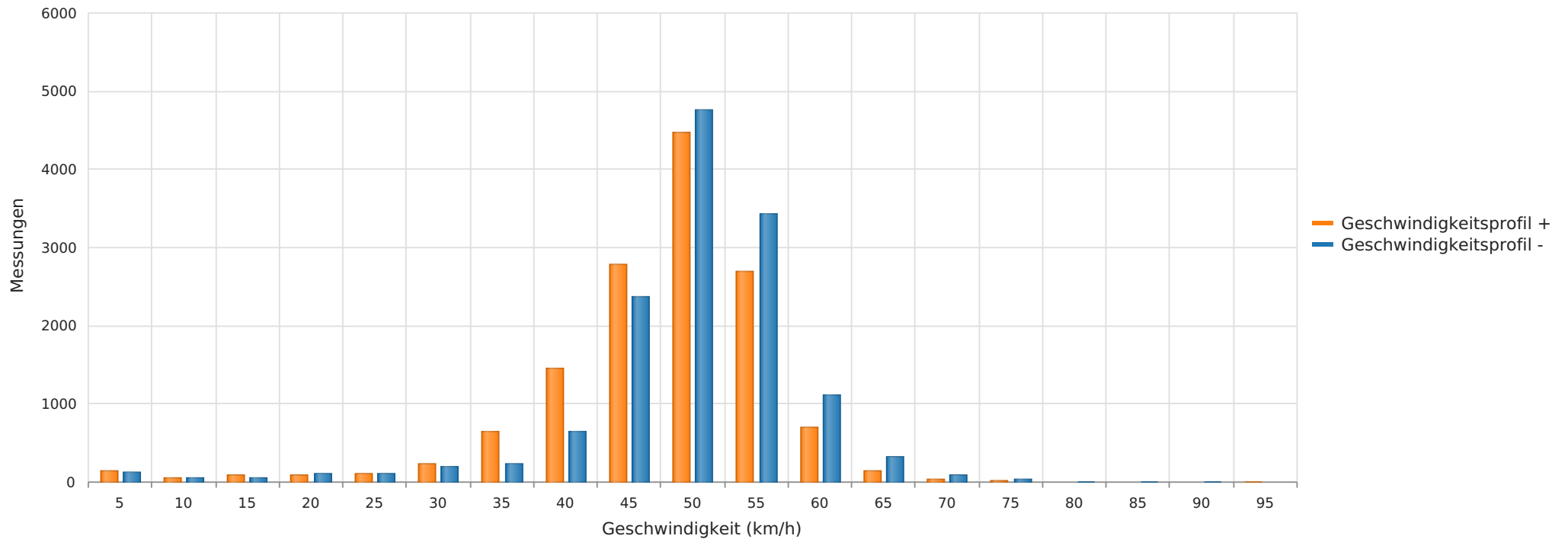
2023_11_12-12_25 Hope Hauptstraße Richtung Grindau Anzahl der Messwerte vs. Geschwindigkeit
